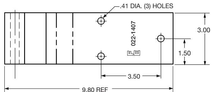
Hinge 022-01407
